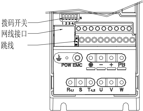
图 3-4 拨码开关和跳线指示图
