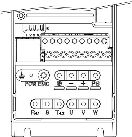
图3-2 G280-4T015GB（15kW）以下主回路端子
