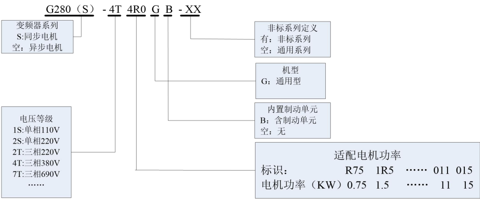
图2-1. 命名规格
