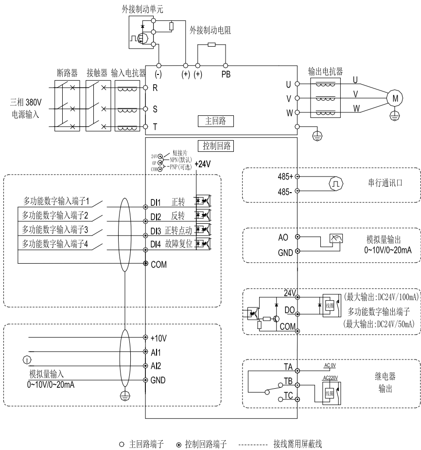
图 3-1. 接线方式（4T:380V）及单相 220V（2S）1.5kW(输入接 L N 或 R T)以下变频器接线图
