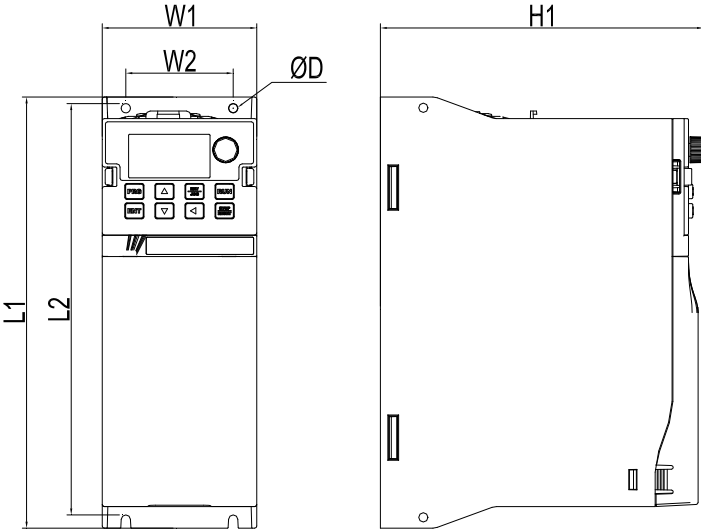
图 2-3. 外观安装尺寸(壁挂式)
