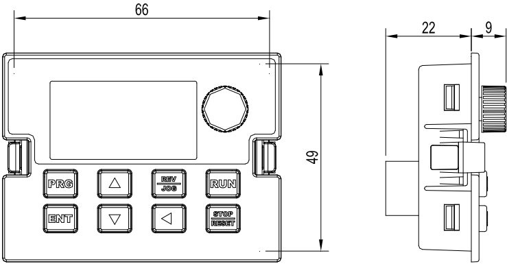
图 2-6 键盘安装开孔尺寸:66×49mm 门板厚度推荐:T=1.2mm
