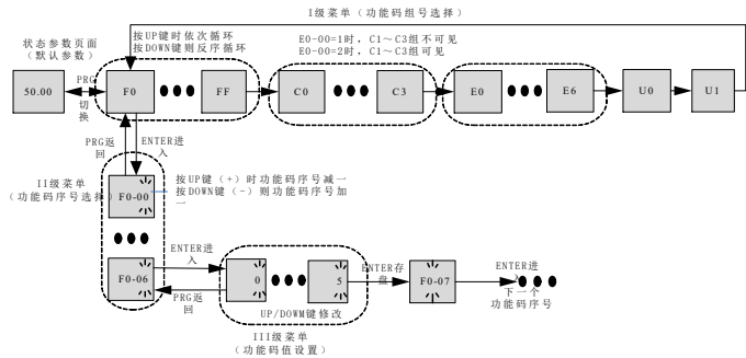
图 4-2. 三级菜单操作流程图
