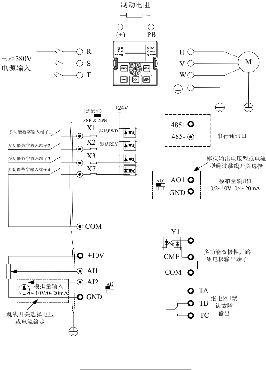
图3-1. 三相380V 2.2kW (4T:380V) 及单相220V (2S) 1.5kW(输入接L N或R T)以下变频器接线图 备注：数字输入端子X跳线开关出厂默认NPN模式（即X短接COM有效），PNP模式为选配功能，三相380V 2.2 kW及单相220V 1.5 kW以下如需选配PNP模式，订货时请说明。AI2,A01跳线开关出厂默认电压模式。
