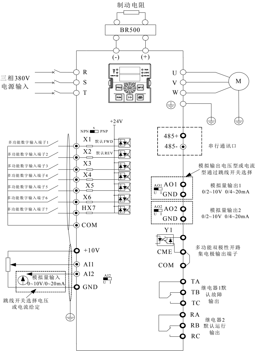
图 3-3. 三相 380V 37 ~ 75 kW (4T:380V) 变频器不带制动单元功能接线图 备注：数字输入端子 X 跳线开关出厂默认 NPN 模式（即 X 短接 COM 有效），AI2、AO1、AO2 跳线开关出厂默认电压模式。G880/G880S 系列 37~110kW 制动单元部分属选配功能，如有需求，订货时请说明，选配了制动单元功能的接线图参考图 3-2。
