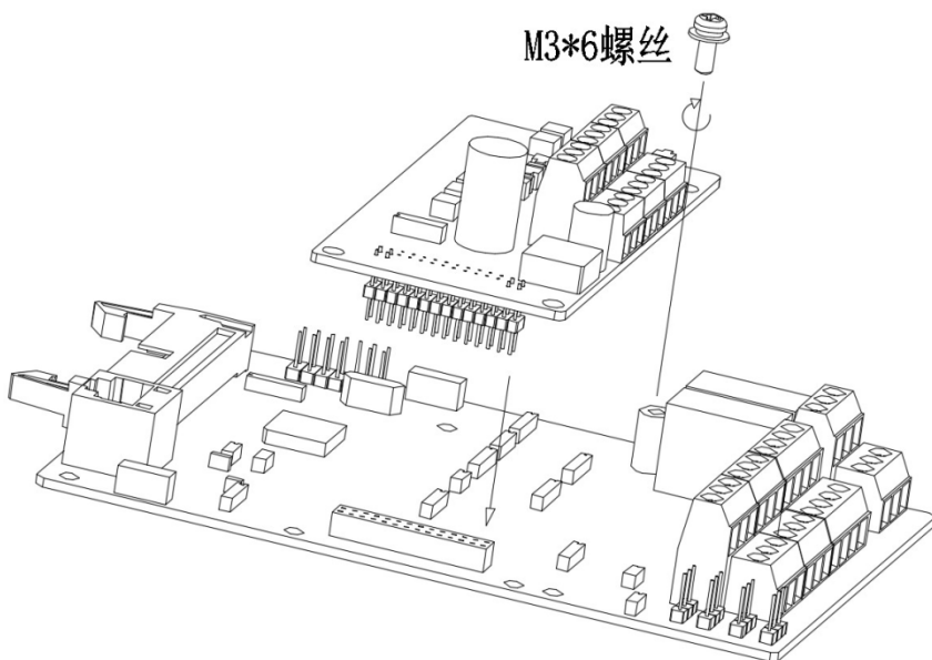
附录 C：图 1 G680/G680S 扩展卡安装方式
