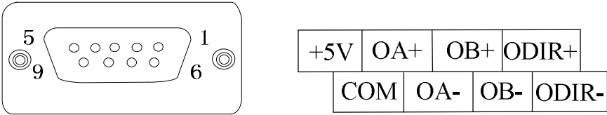
附录 B：图 5 G680-PGR 端子图
