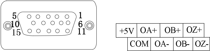
附录 B：图 7 G680-PGS 端子图
